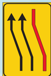
FIG. 412/e ART. 43 SEGNALE DI RIENTRO IN CARREGGIATA
